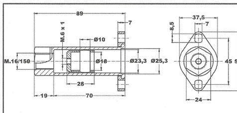
CONEXION DISTRIBUIDOR 1/2" KIT 002
