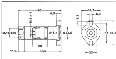
CONEXION DISTRIBUIDOR 3/8" KIT 001
