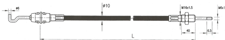
Cable tipo 6010/17-1
